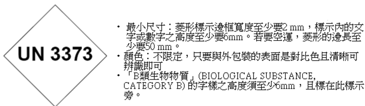
圖十、運送 B 類感染性物質的標示
